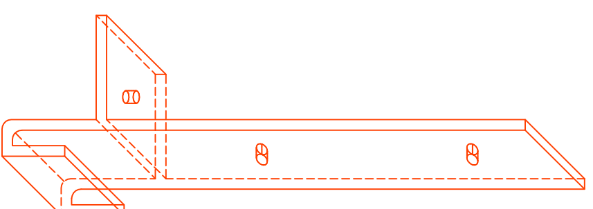
IZOMETRIJA JEKLENI PROFIL Z OZNAKO 1
