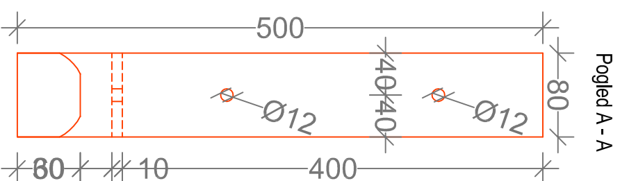
Jekleni profil oznaka 1 40 kom M 1:10
