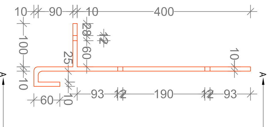
Jekleni profil oznaka 1 40 kom M 1:10
